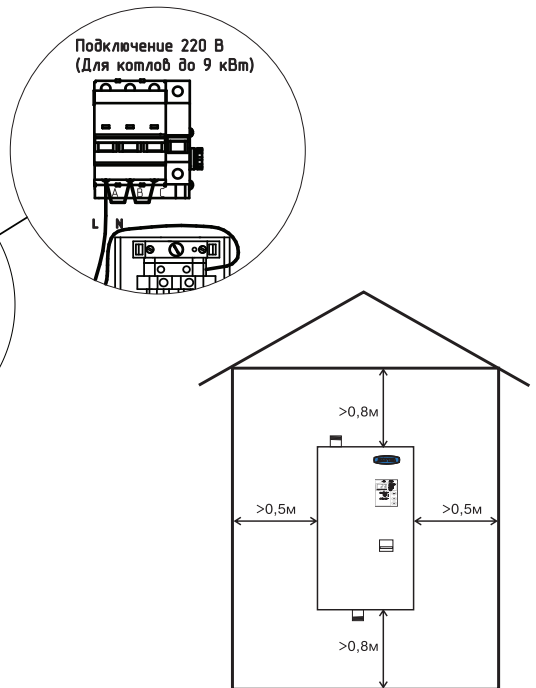
Рис. 4 Схема установки электроводонагревателя
